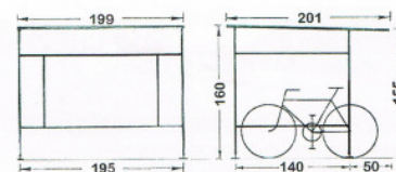
„Garden Light“ Front- u. Seitenansicht - Traufe vorn
